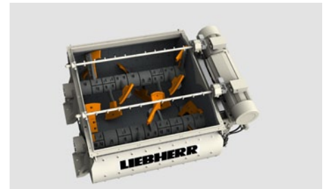
Doppelwellenmischer einer Betonmischanlage, gerendert mit KeyShot
